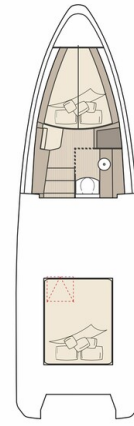
Saxdor 340 WA lower layout
