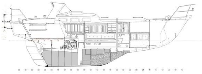
REKERE 36 msp794769 Langsschnitt
